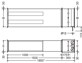
Type NKOF0RB (retour)
