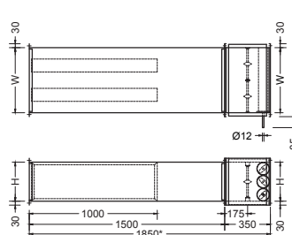
Type NLOFORB (retour)
